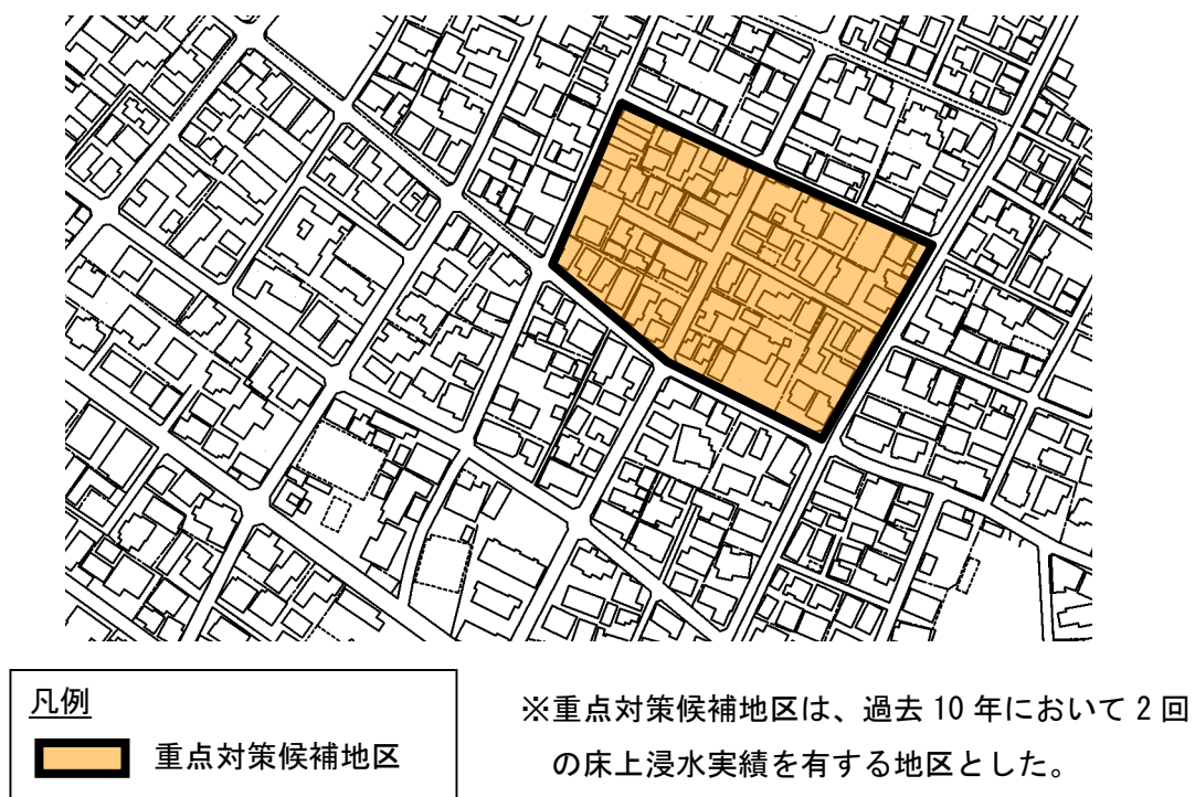
図3-6 カテゴリーCにおける重点対策候補地区（浸水常襲地区）の設定例
