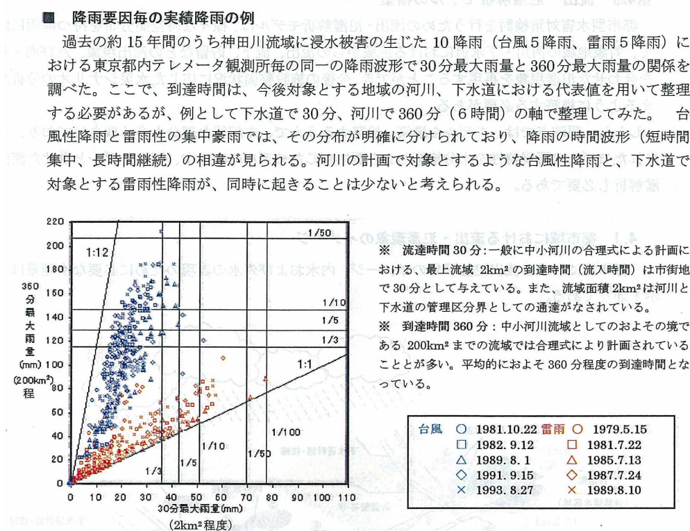
図2-2 降雨要因毎の実績降雨の例（東京都内のテレメータ雨量）
