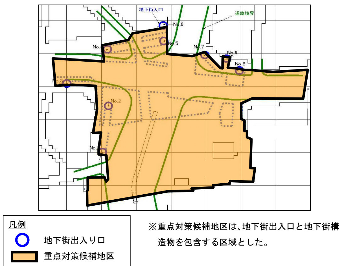
図3-4 カテゴリーAにおける重点対策候補地区（高度地下空間利用地区）の設定例
