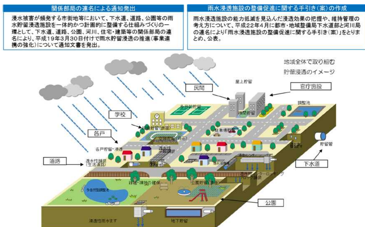
図7-2 流域全体で取り組む貯留浸透のイメージ
