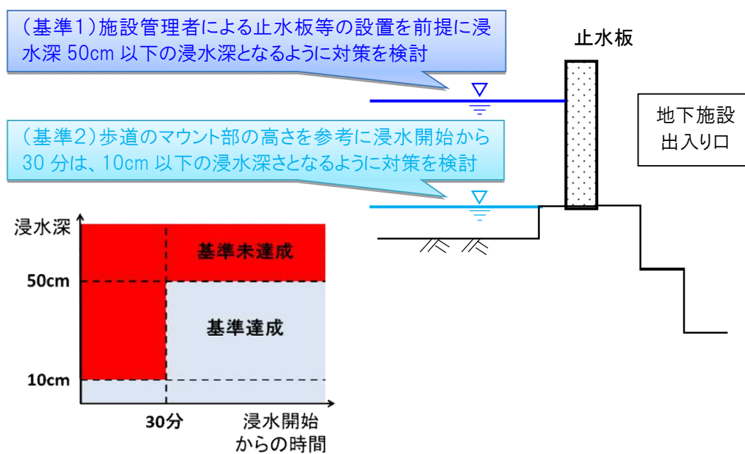
図3-9 地下施設の出入口付近における機能保全水深と浸水開始時間の設定例
