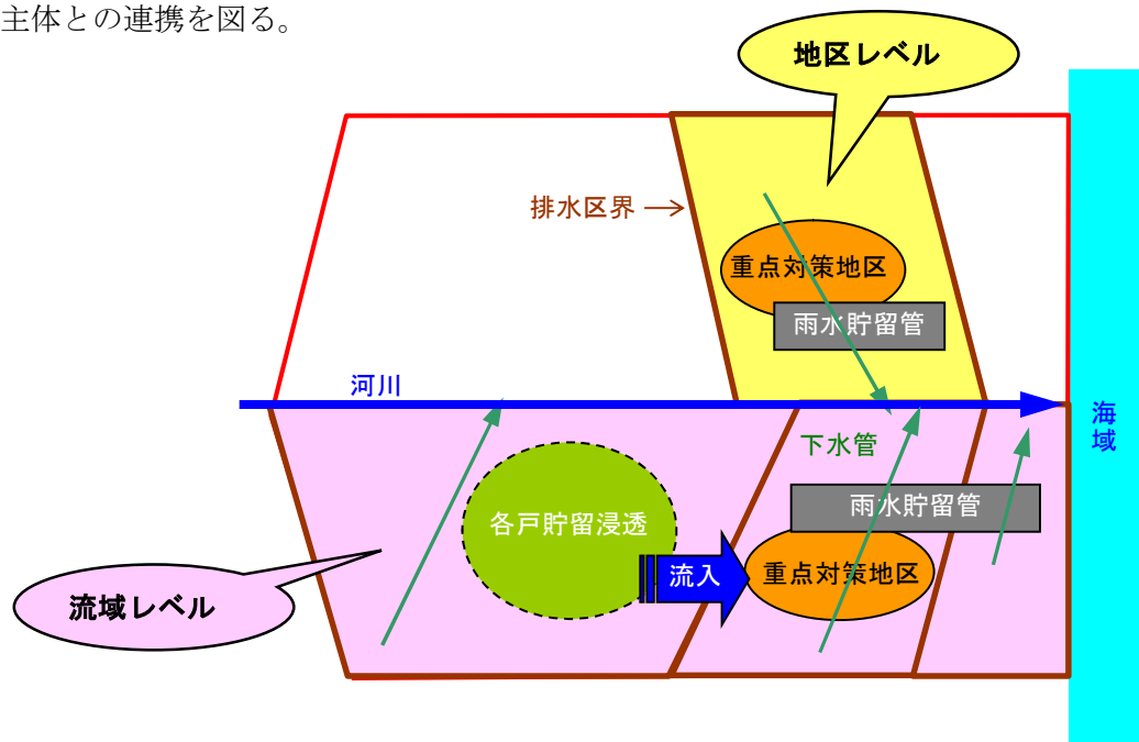
図 7-4 地区レベル及び流域レベルのイメージ
