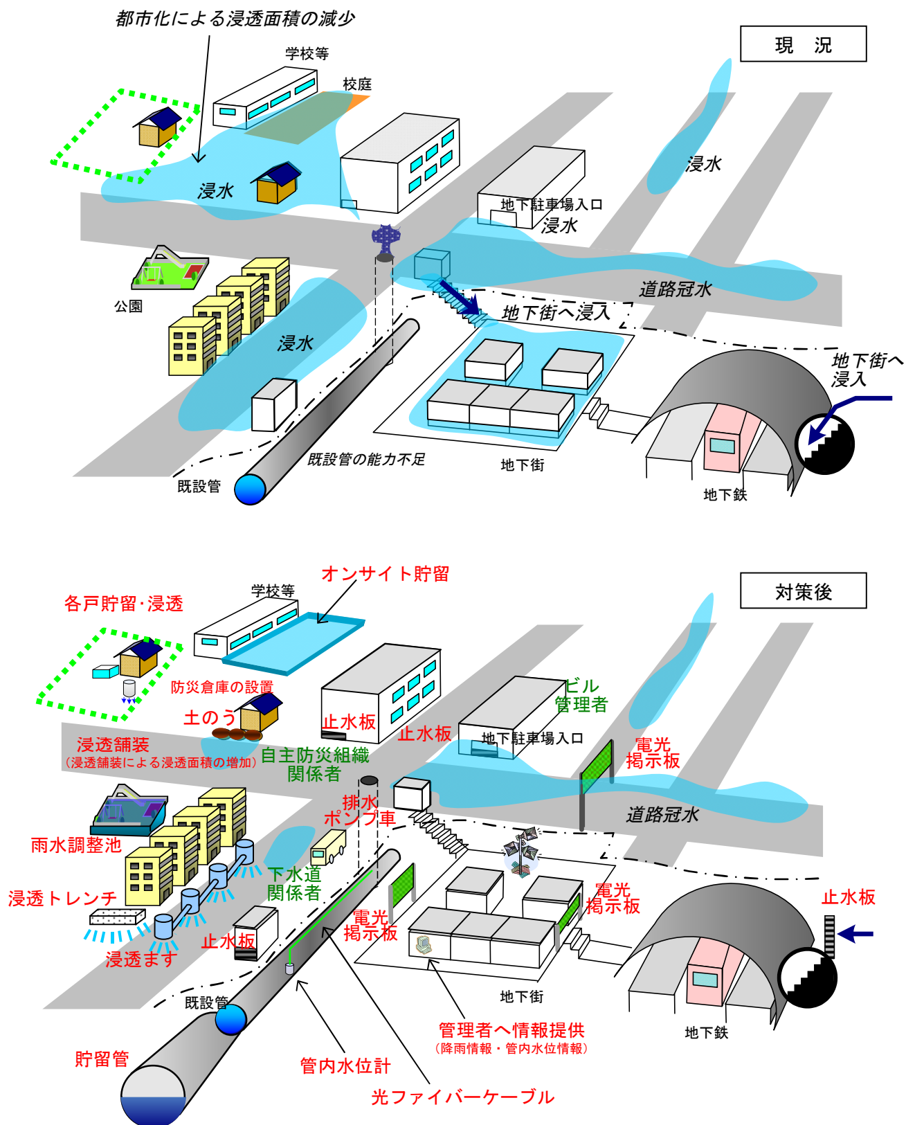
図5-10 総合的な浸水対策のイメージ
