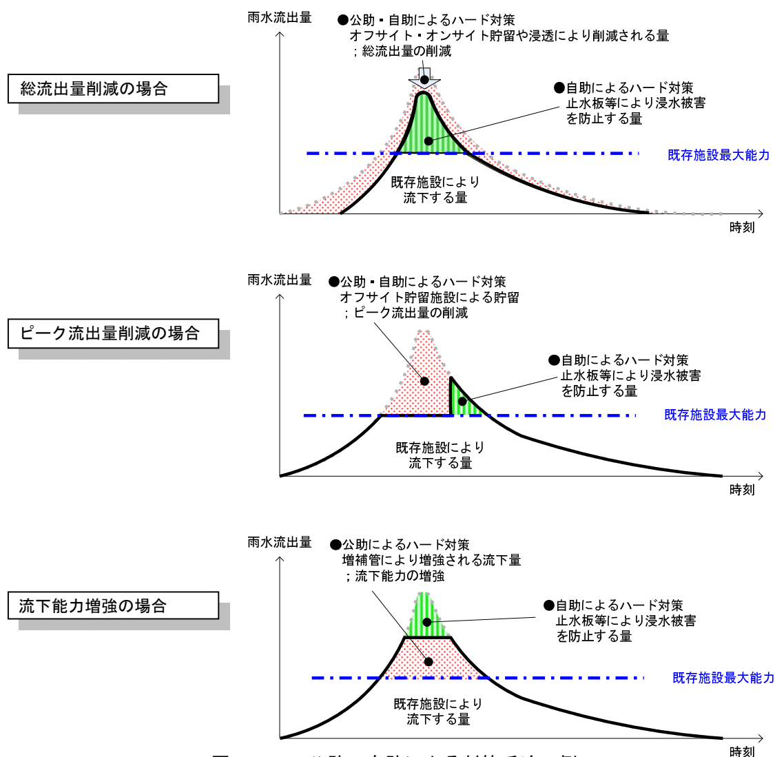
図5-4 公助・自助による対策手法の例
