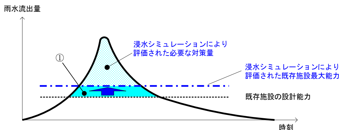
図5-3 既存施設の能力評価
