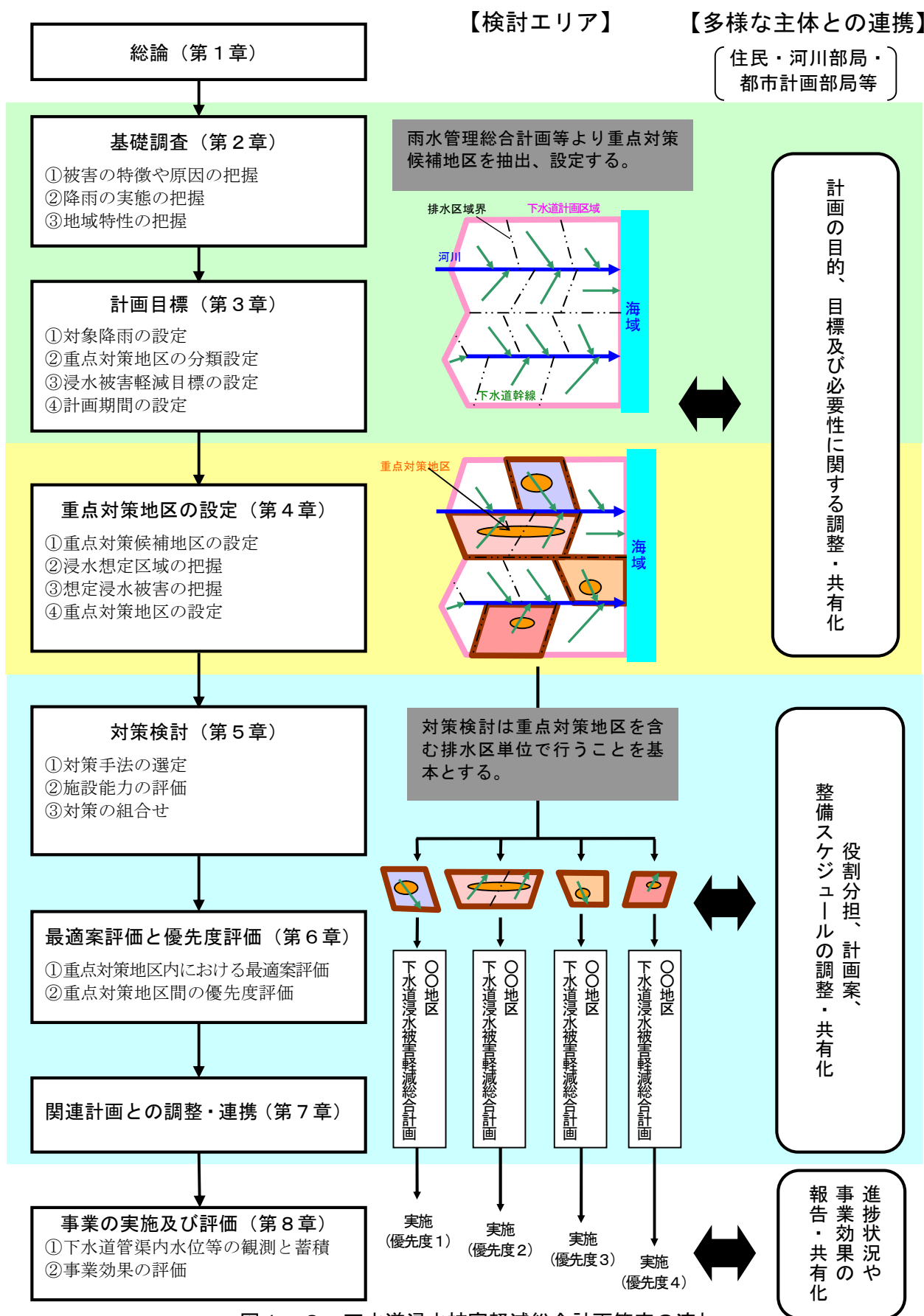
図1-8 下水道浸水被害軽減総合計画策定の流れ
