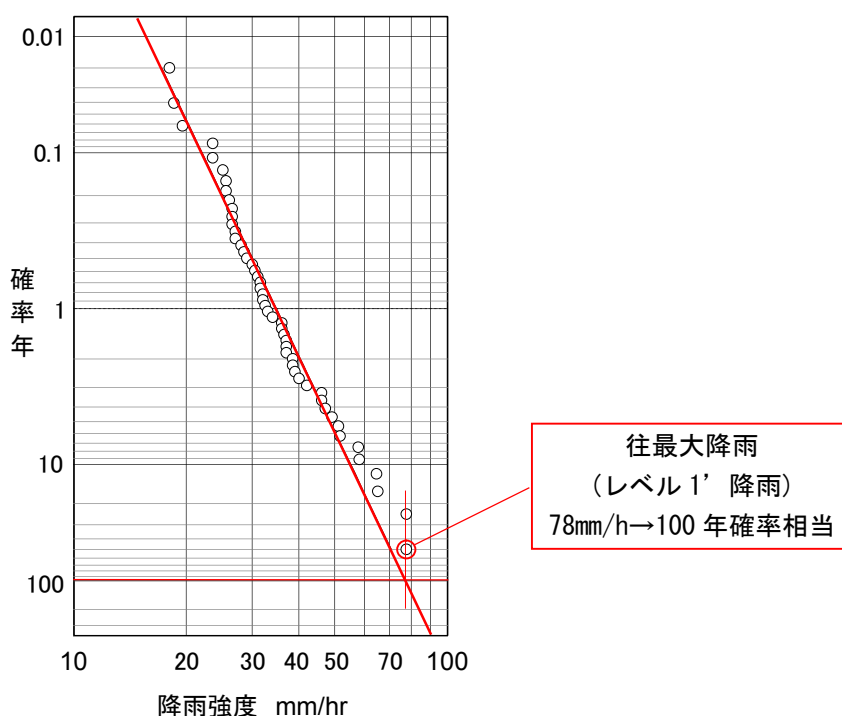
図 6-2 実績降雨の確率評価のイメージ
