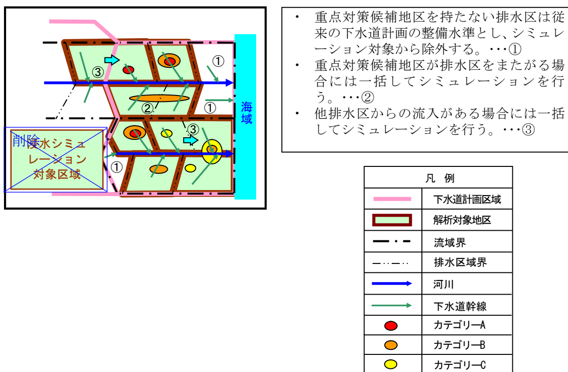
図 4－4 現況施設の浸水シミュレーションにおける対象区域のイメージ
